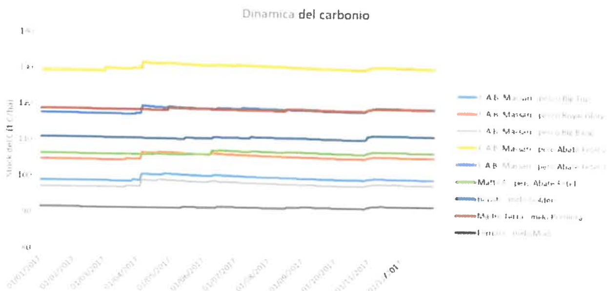
Fig. 4 - Risultati della simulazione della dinamica di C nel suolo secondo il modello DNDC
